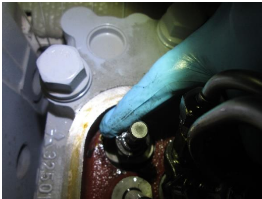
Inspección de cabeza del motor (cilindro 12)
