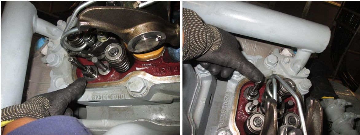
La válvula sufrió rotura en la cabeza, el vástago quedó suelto.
